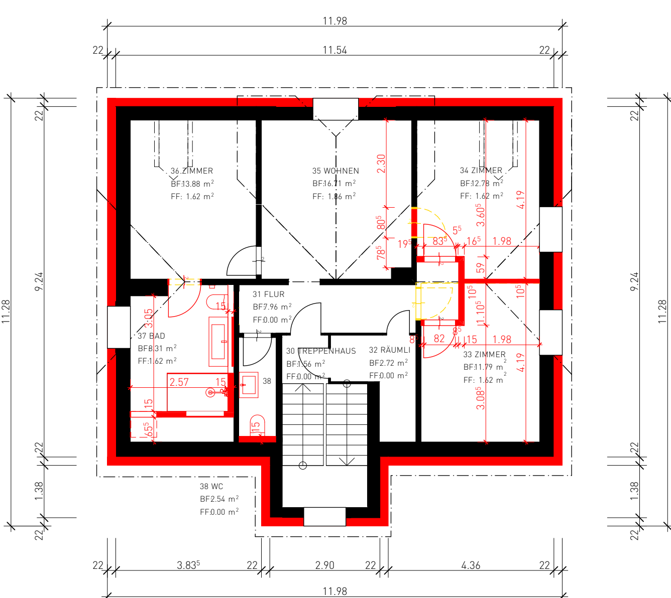
GRUNDRISS 2.OG MST. 1:100
