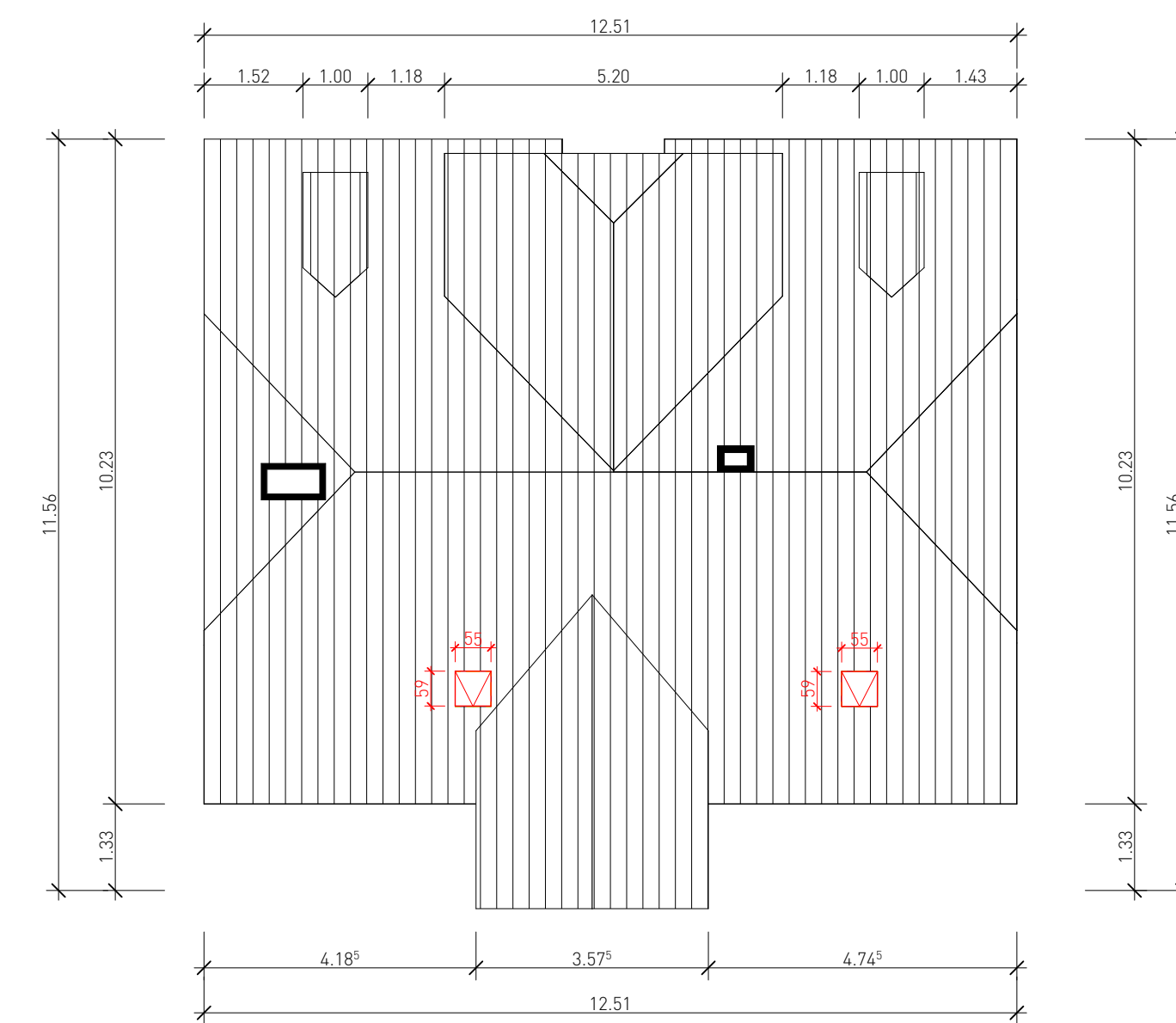
DACHAUFSICHT MST. 1:100
