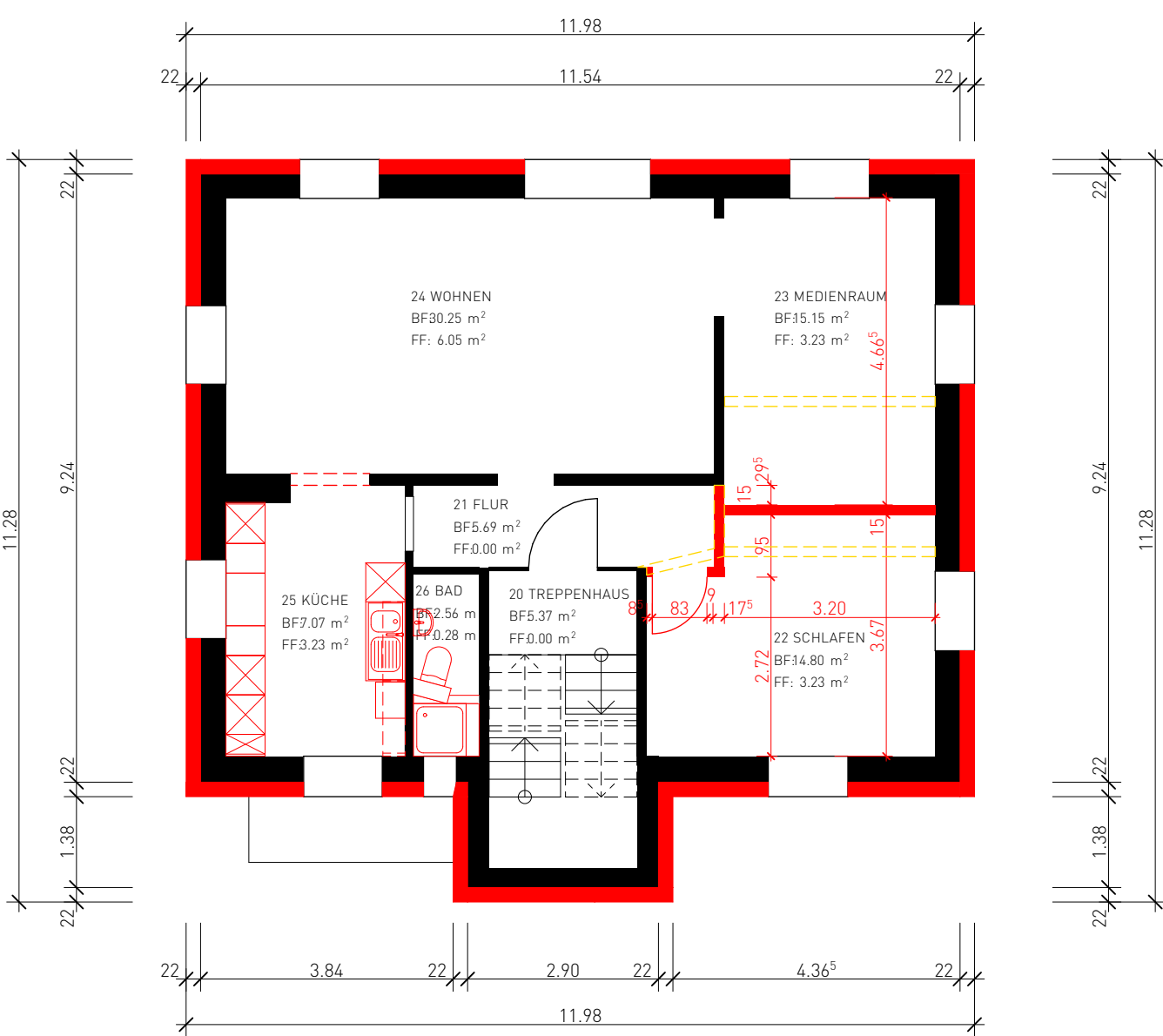
GRUNDRISS 1.OG MST. 1:100
