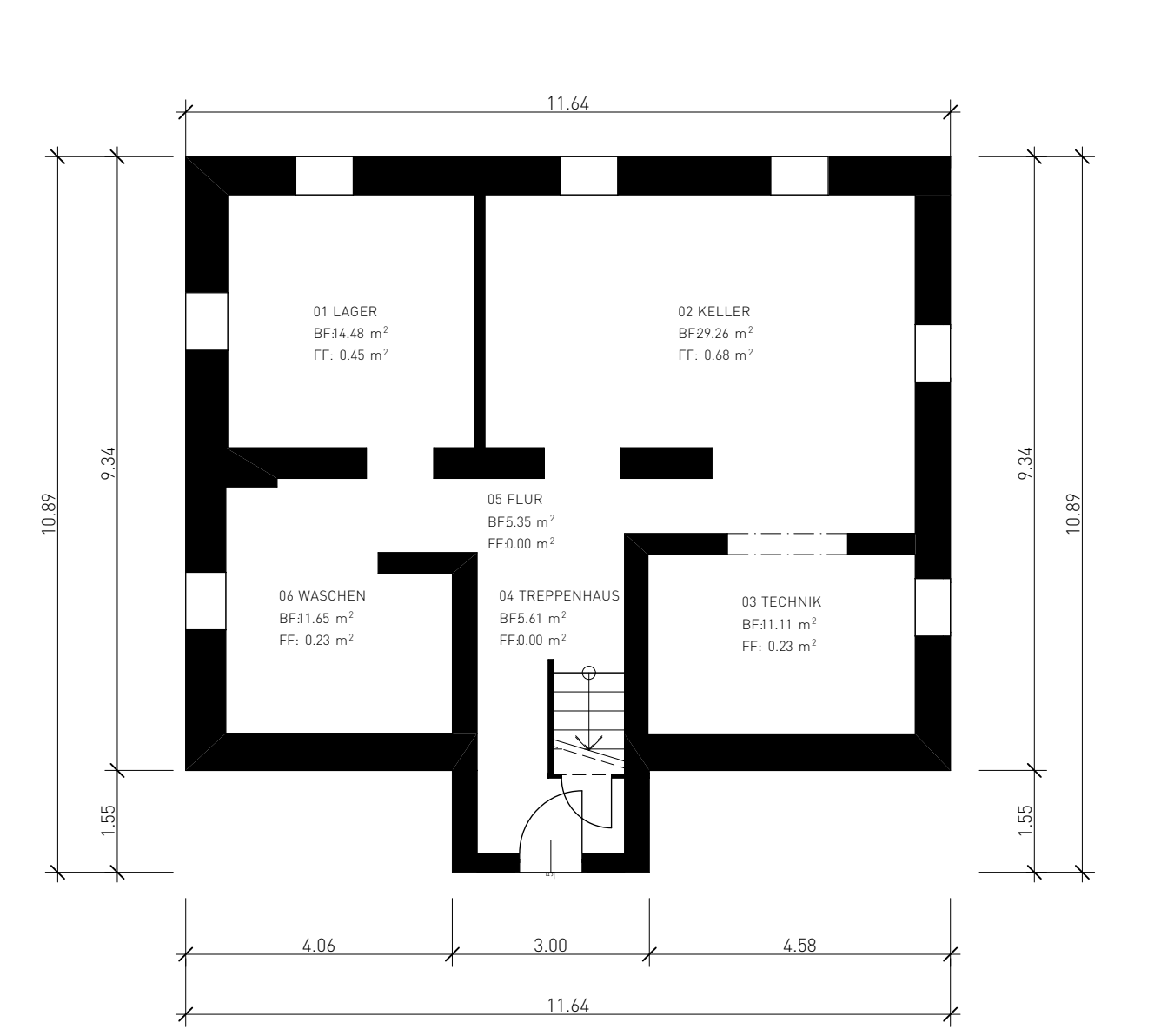
GRUNDRISS UG MST. 1:100
