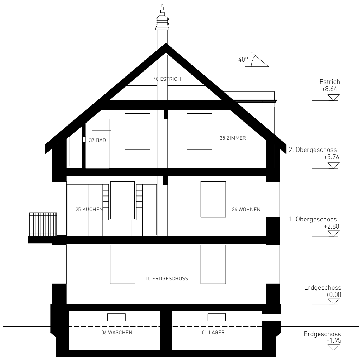
SCHNITT MST. 1:100
