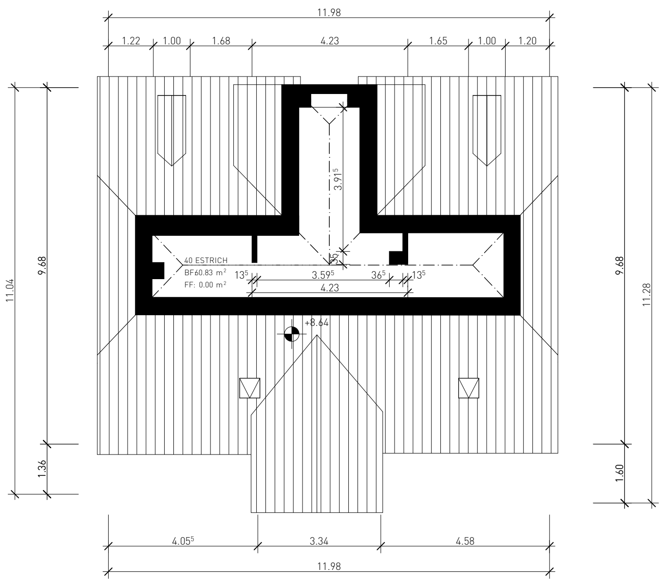
GRUNDRISS DG MST. 1:100
