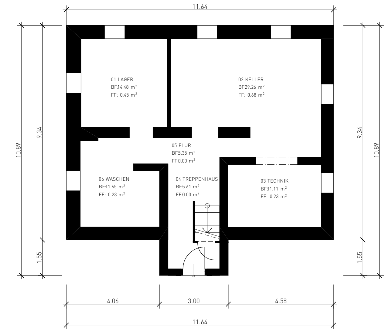
GRUNDRISS UG MST. 1:100
