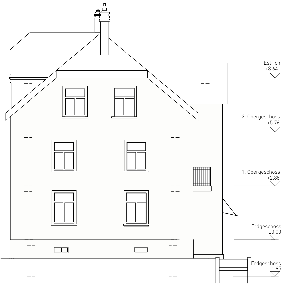
WESTFASSADE MST. 1:100
