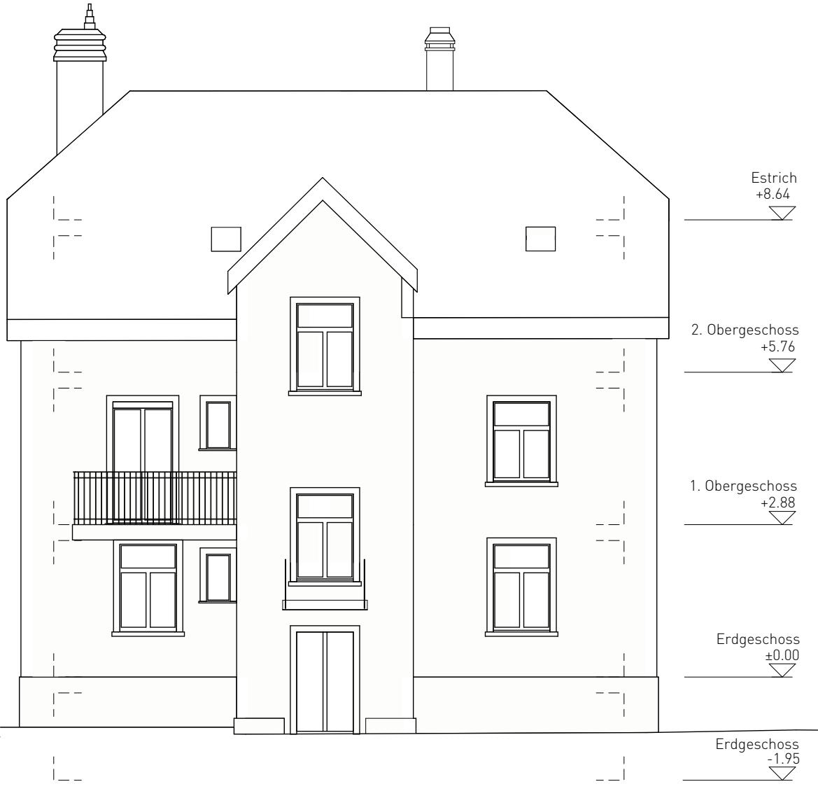
SÜDFASSADE MST. 1:100
