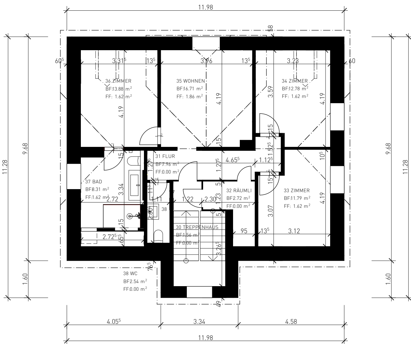
GRUNDRISS 2.OG MST. 1:100
