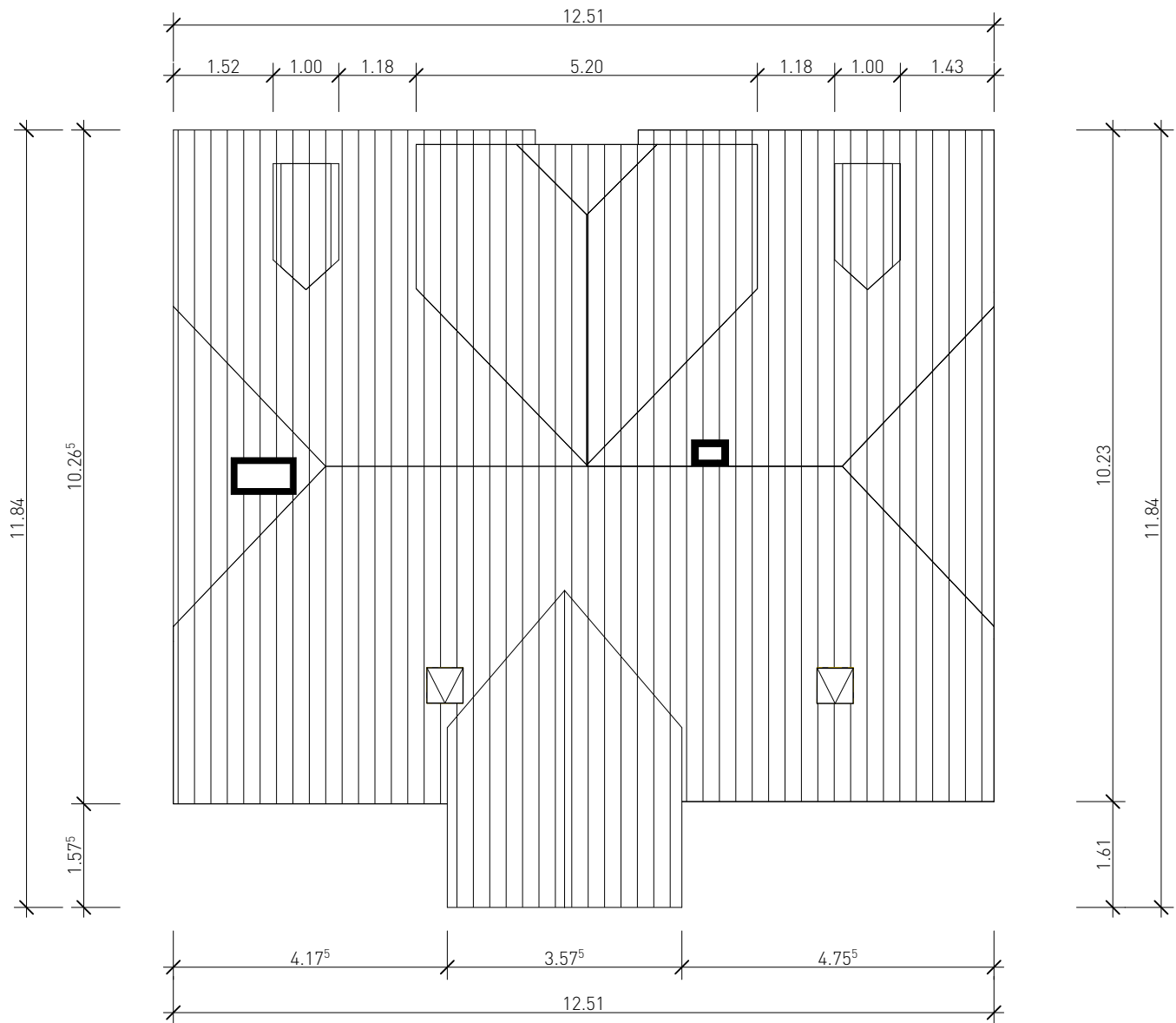
DACHAUFSICHT MST. 1:100
