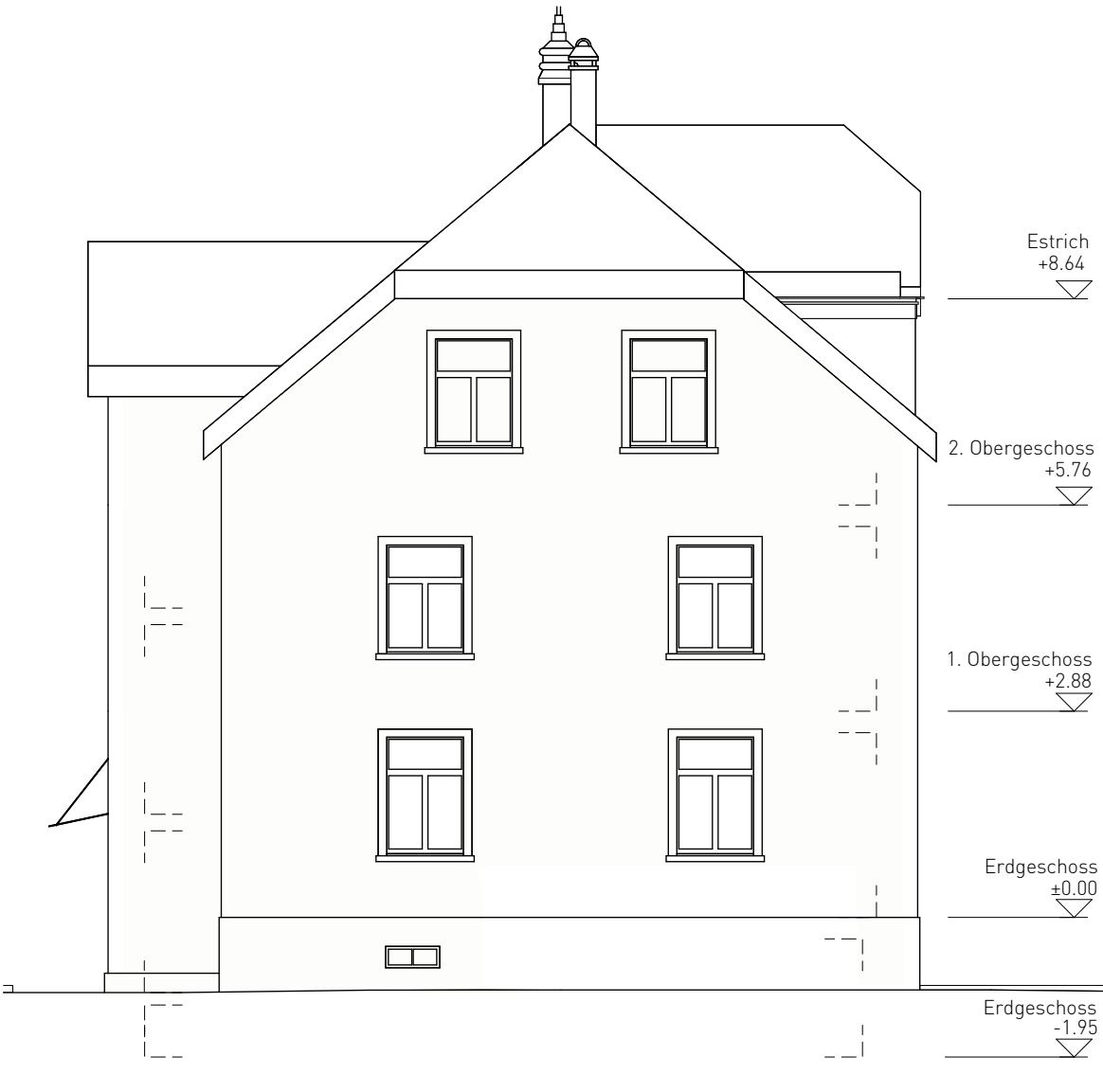
OSTFASSADE MST. 1:100
