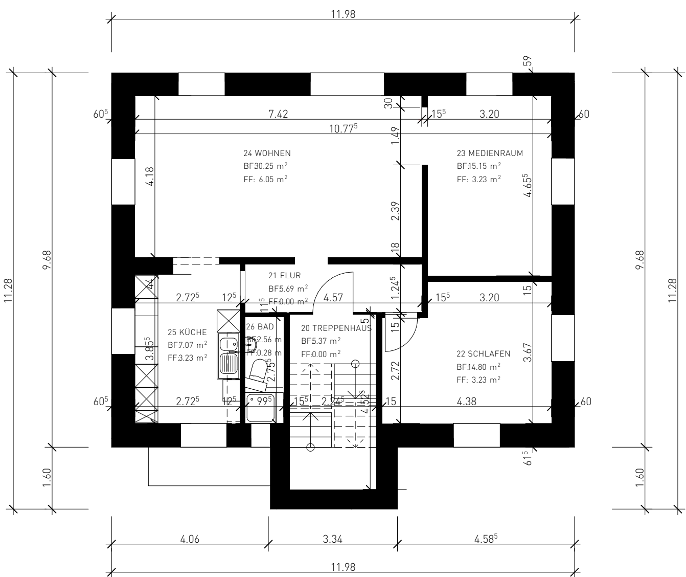
GRUNDRISS 1.OG MST. 1:100
